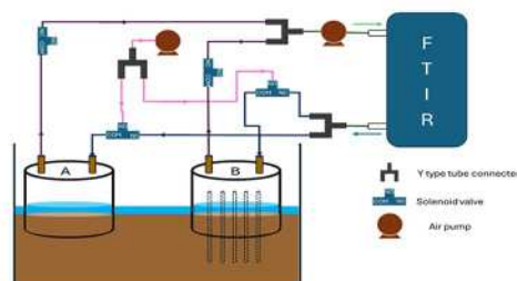
Fig. 1-1 ガス測定システムの概要
