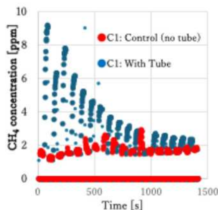
Fig. 1-2 ガス透過性チューブの有無によるチャンバー内の CH 4 濃度変化の違い
