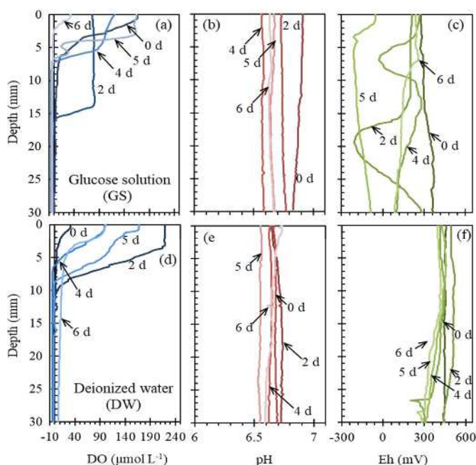
Fig.3-2 水分浸透開始 6 日間のカラム表層 30 mm の溶存酸素濃度 (DO), pH, 酸化還元電位 (Eh) の鉛直分布。上段 ((a)~(c)) は GS, 下段 ((d)~(f)) は DW の分布
