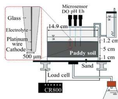
Fig. 3-1 湛水土カラム実験の概略
