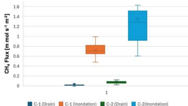
Fig.3-4 酸性泥炭(C-1)と中性泥炭(C-2)の排水時および湛水時の CH 4 フラックスの比較
