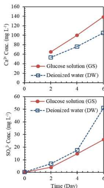
Fig.3-3 水分浸透開始 6 日間のカラム下端流出液中の \text{Ca}^{2+} および \text{SO}_4^{2-} 濃度
